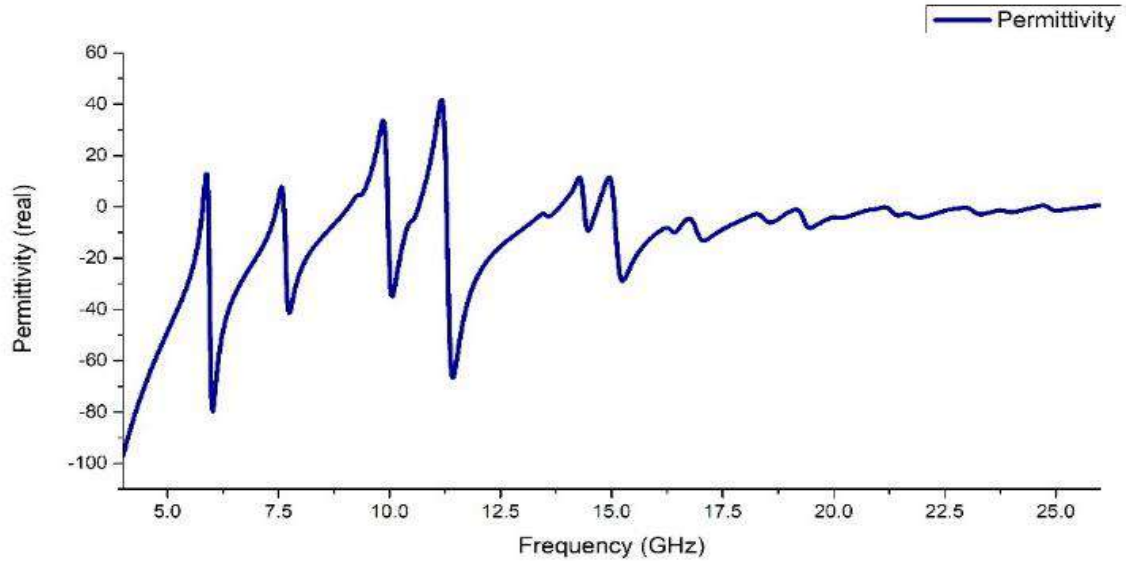
Fig 4.6: Permittivity(real)
