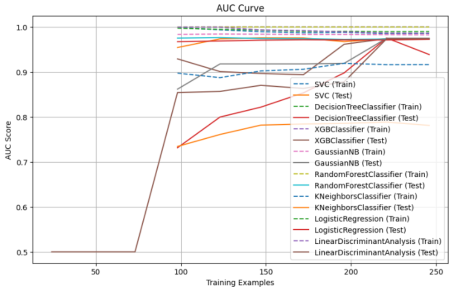
Fig. 4.17. AUC Curve
