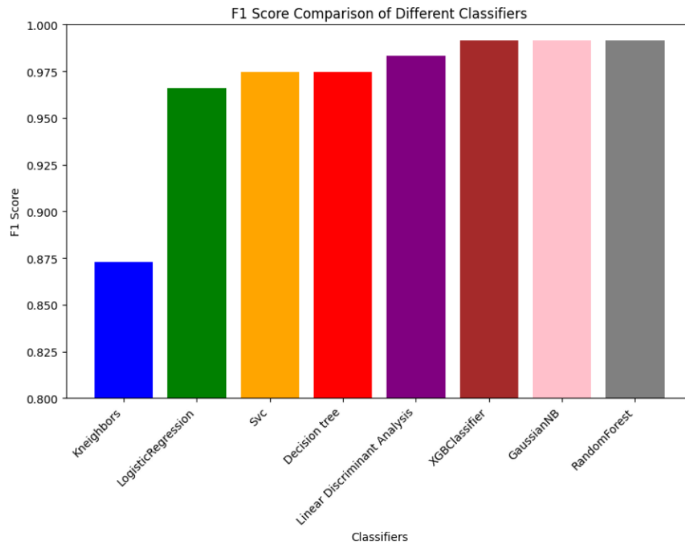
Fig. 4.14. F1 score comparison of different classifiers
