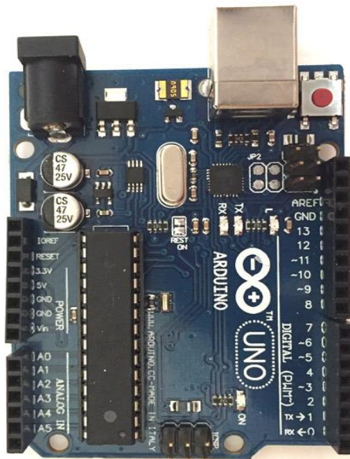
Figure 3 Arduino UNO [24]
